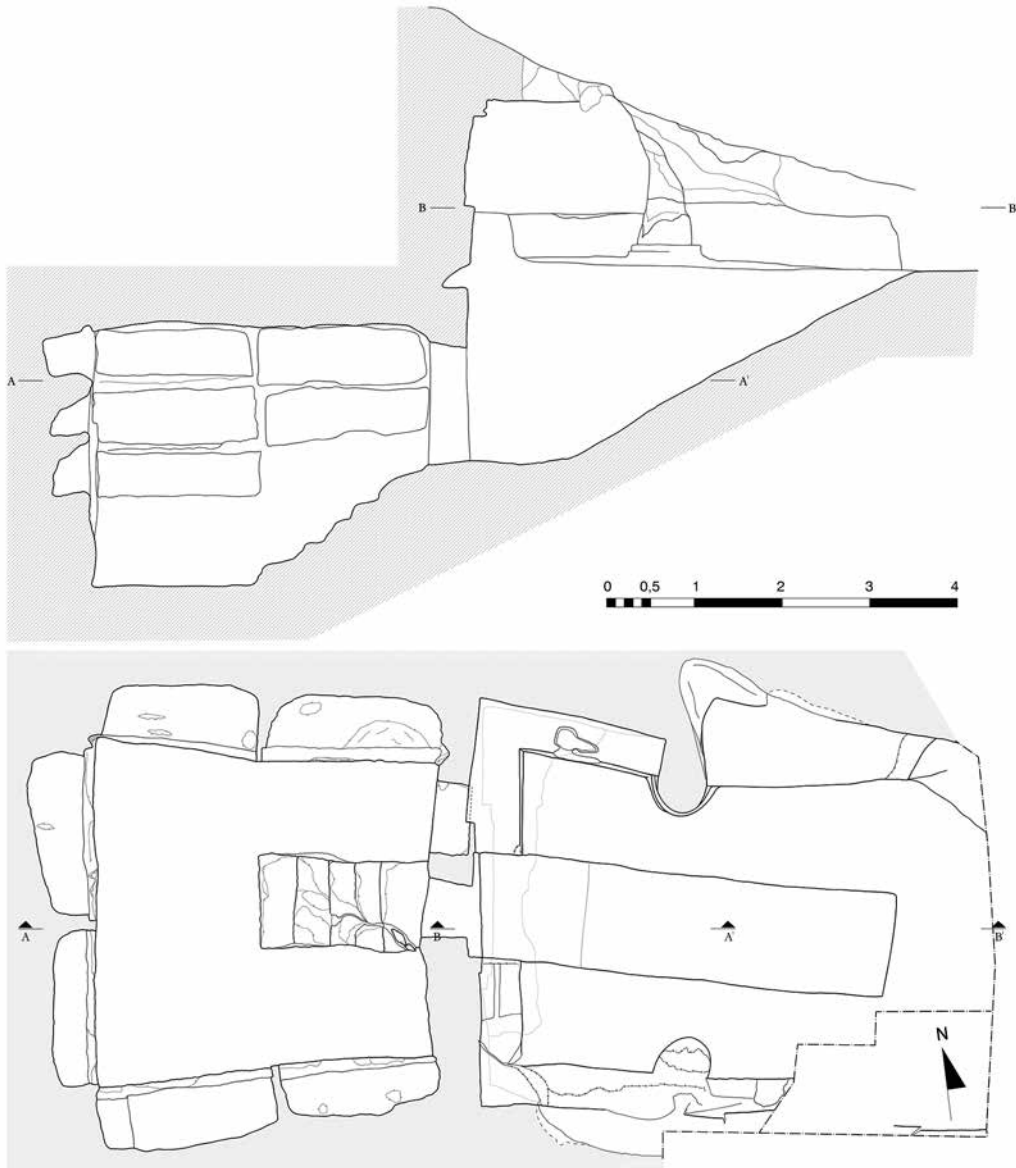
fig. 10 - Tomba n. 10 in loc. Genitura, II, pianta e sezione.
