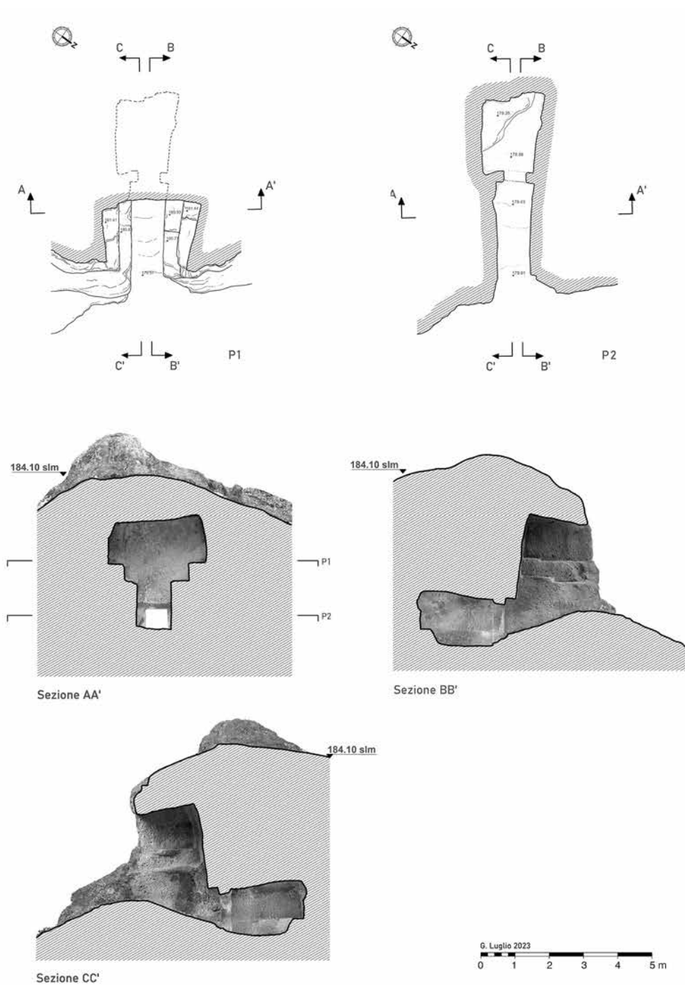
fig. 14 - Tomba n. 14 in loc. Pastine, I, pianta e sezione.
