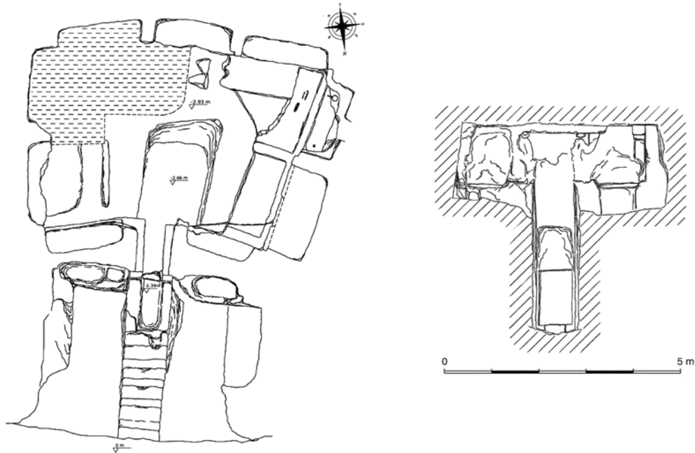
fig. 11 - Tomba n. 11 in loc. Vallecchia, I, pianta e prospetto.
