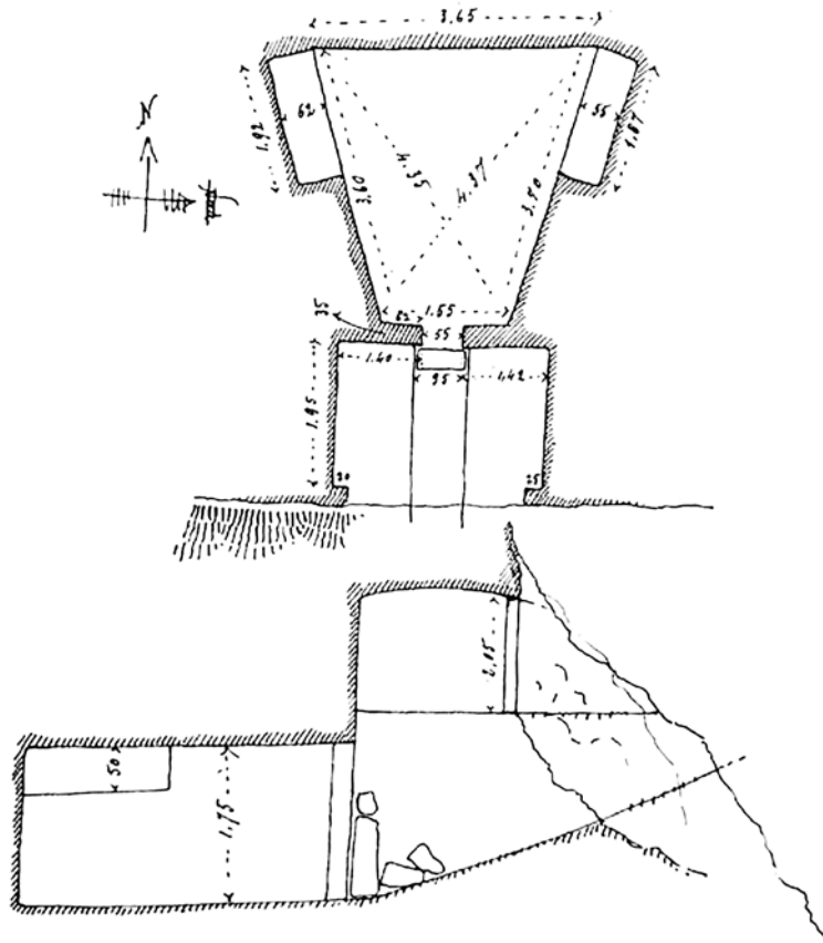
fig. 7 - Tomba n. 7 in loc. Fustignano, schizzo misurato.
