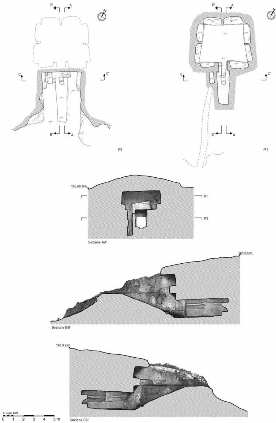
fig. 16 - Tomba n. 16 in loc. Valspigliaro, pianta e sezione.
