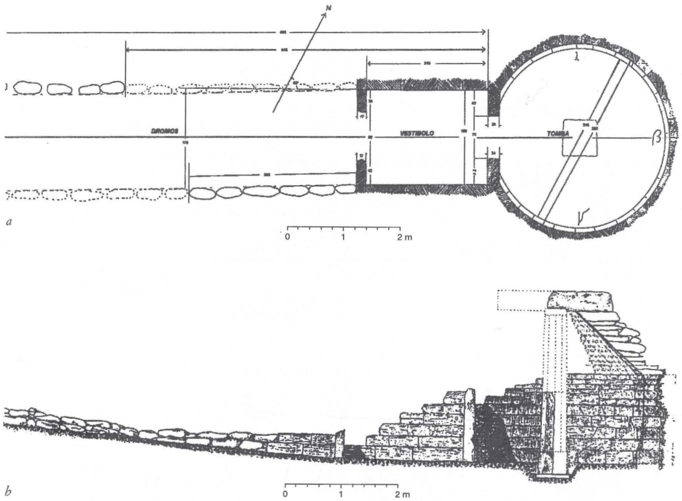
fig. 6 - a-b) Volterra, tomba di Casaglia: pianta e sezione.
