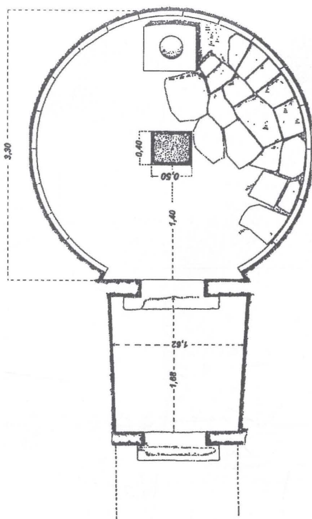
fig. 4 - Casale Marittimo, tomba a tholos : pianta.
