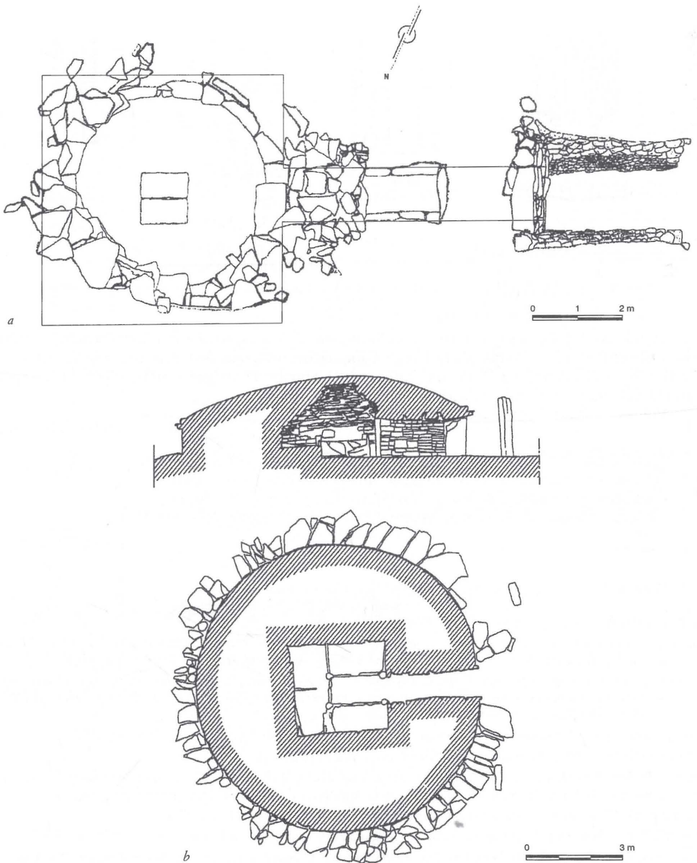
fig. 13 - a) Vetulonia, tomba del Diavolino 2: pianta; b) Populonia, tomba dei Flabelli: sezione e pianta.
