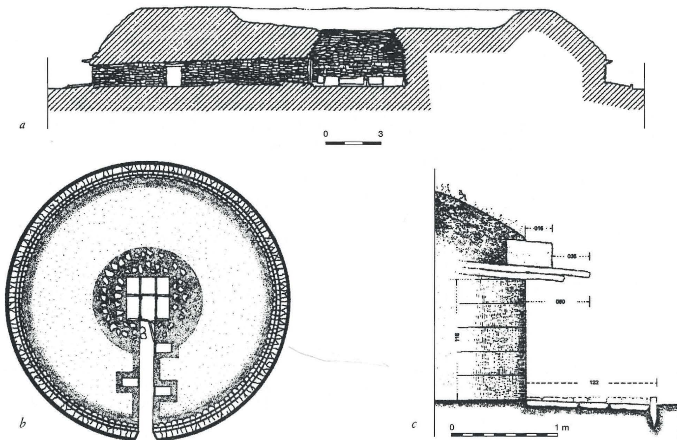
fig. 3 - a-c) Populonia, tomba dei Carri: sezione, pianta e sezione della krepis .
