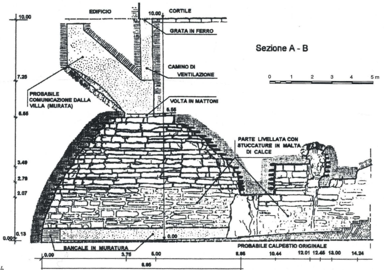
fig. 8 - a-b) Quinto Fiorentino, tomba della Mula: pianta e sezione.
