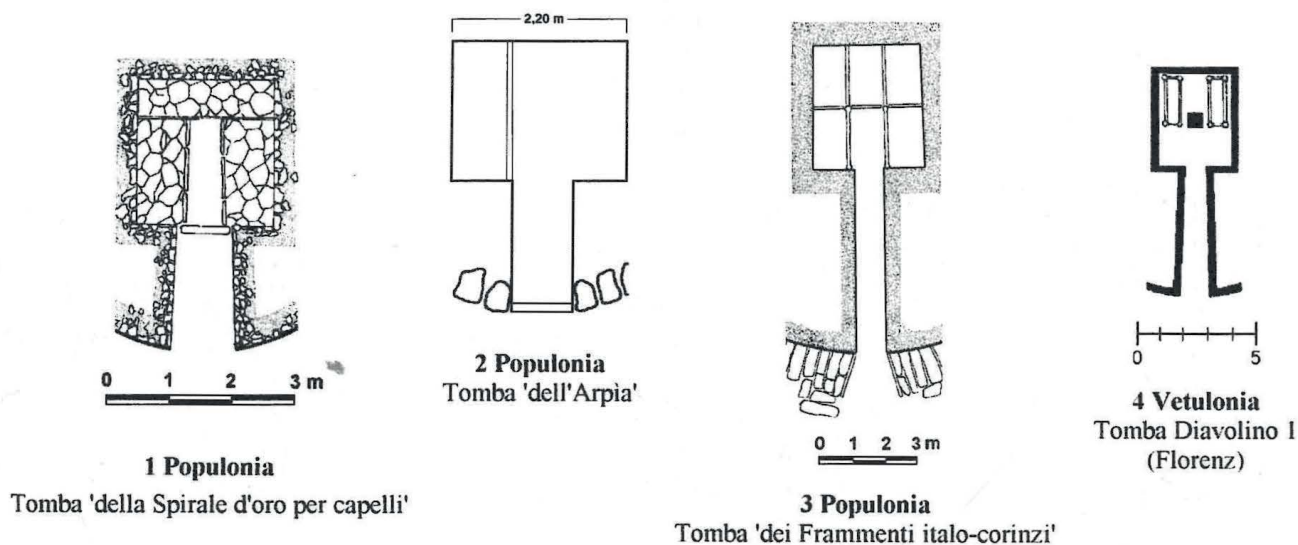
fig. 12 - Piante di tombe etrusche a cupola con pianta rettangolare.
