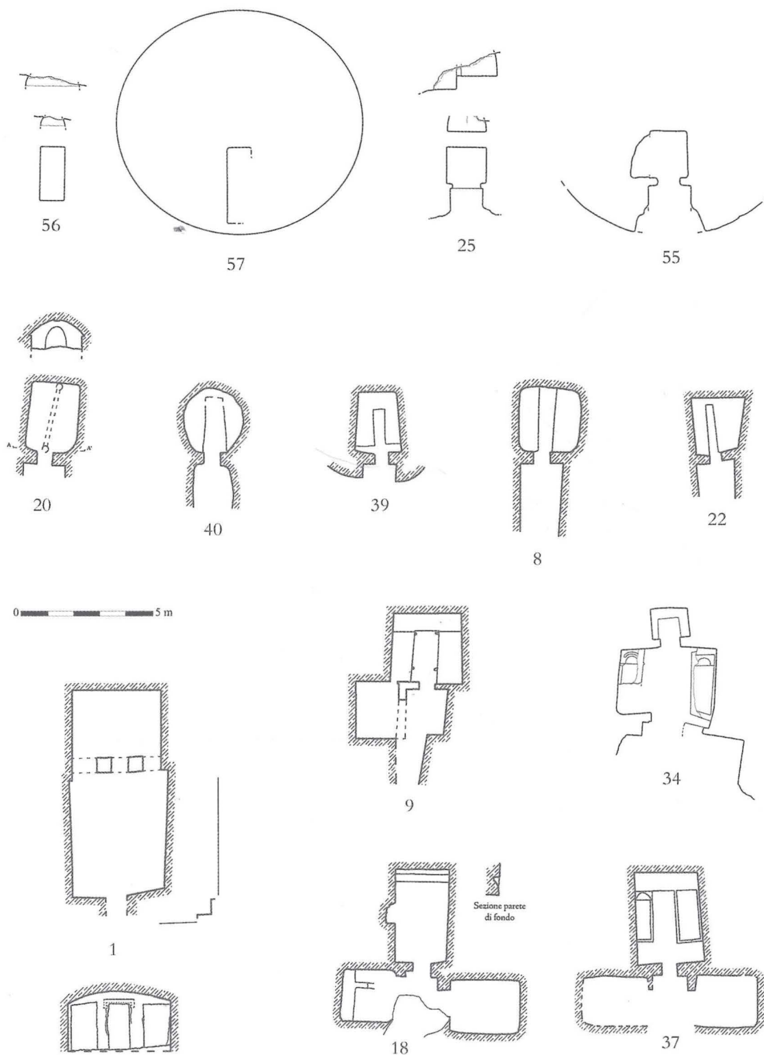
fig. 4 - Necropoli di Largo della Bandita, piante delle tombe nn. 1 "Grotta di Tabacco", 8, 9, 18, 20, 22, 25, 34, 37, 39, 40, 55, 56, 57.
